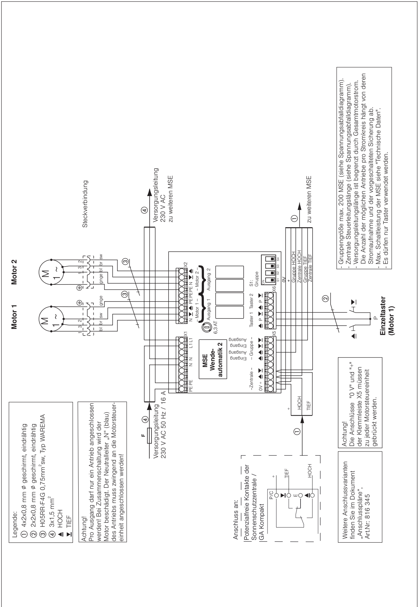
Abb. 5 Anschlussplan MSE Wendeautomatik 2 AP und REG
