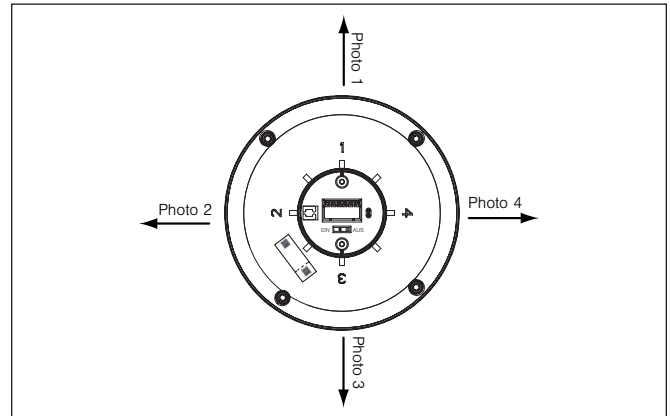
Abb. 3 Position der Photodioden am Gerät
