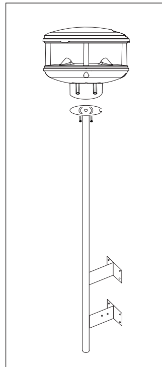
Abb. 4 Wandmontage auf Standrohr
