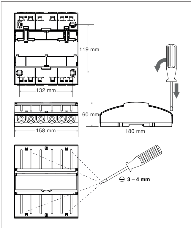
Abb. 4 Abmessungen AP-Gehäuse
