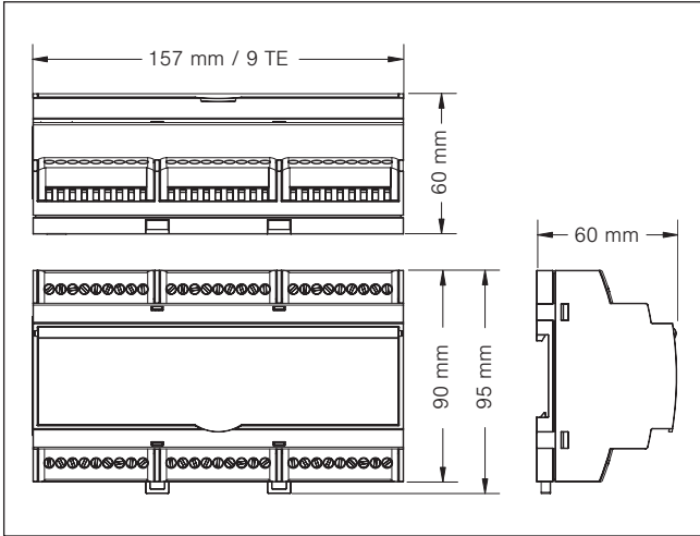
Abb. 2 Abmessungen REG-Gehäuse
