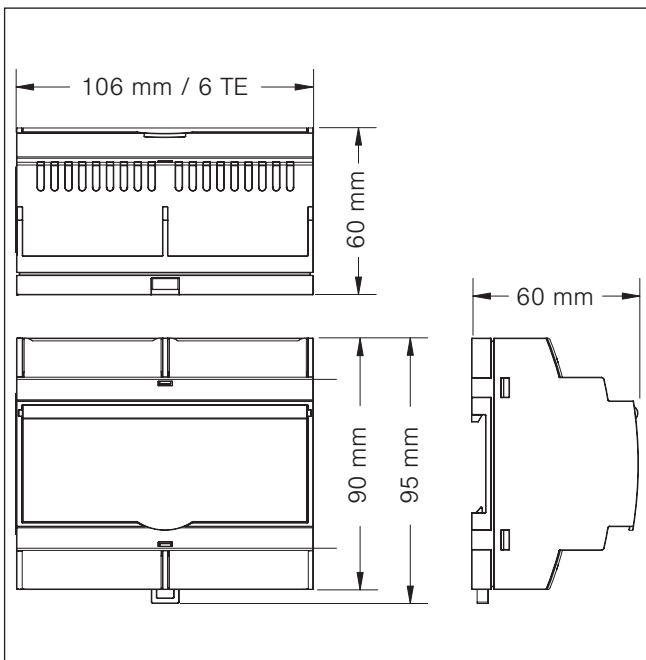
Abb. 3 REG-Gehäuse 6 TE für MSE Kompakt 6
