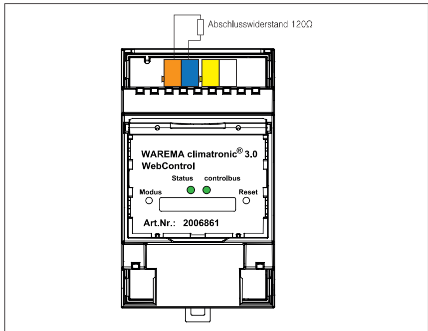
Abb. 25 Reset-Taste zum Laden der Firmware
