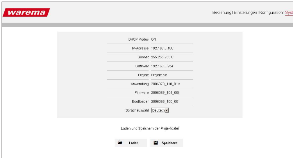
Abb. 24 Statusinformationen des Menüpunkts "System".
