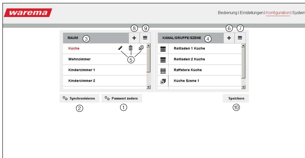
Abb. 7 Oberfläche des WAREMA climatronic® WebControl, Menü Konfiguration
