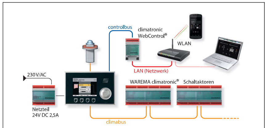
Abb. 2 Anschluss des WAREMA climatronic® WebControl
