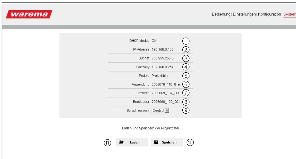
Abb. 9 Oberfläche des WAREMA climatronic® WebControl, Menü "System"
