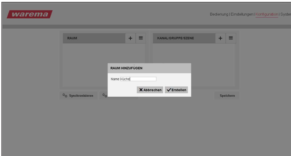
Abb. 14 Räume erstellen
