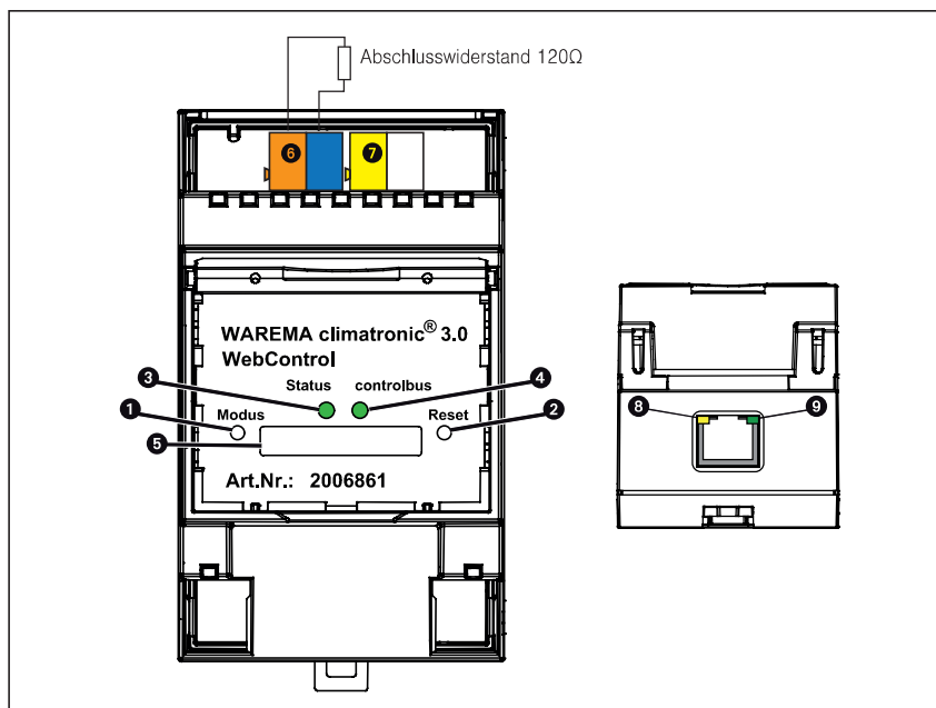
Abb. 4 Anschlüsse und LEDs des WAREMA climatronic® WebControl (Vorderansicht, Unterseite)
