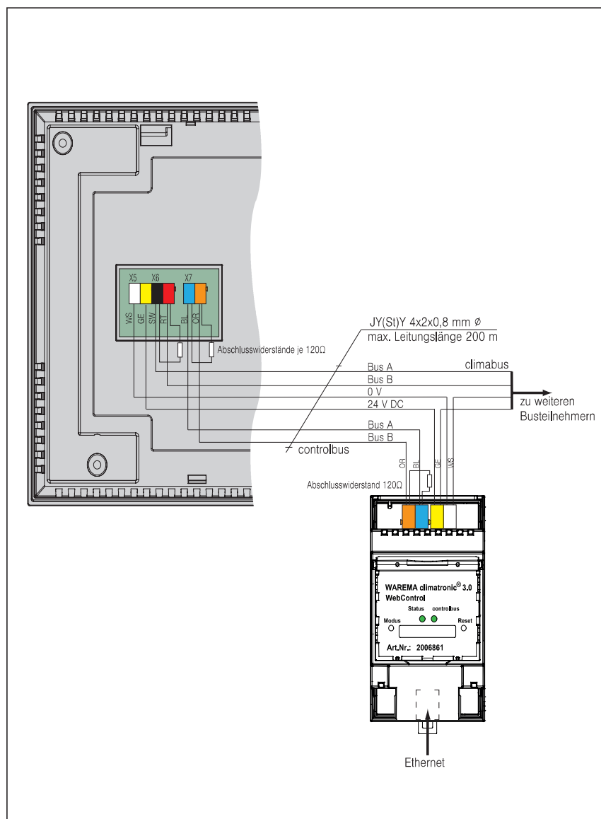
Abb. 3 Anschlussplan
