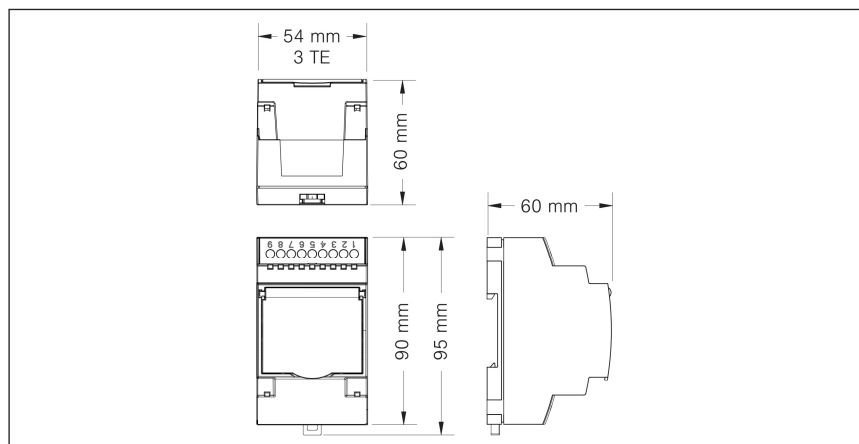
Abb. 27 Abmessungen
