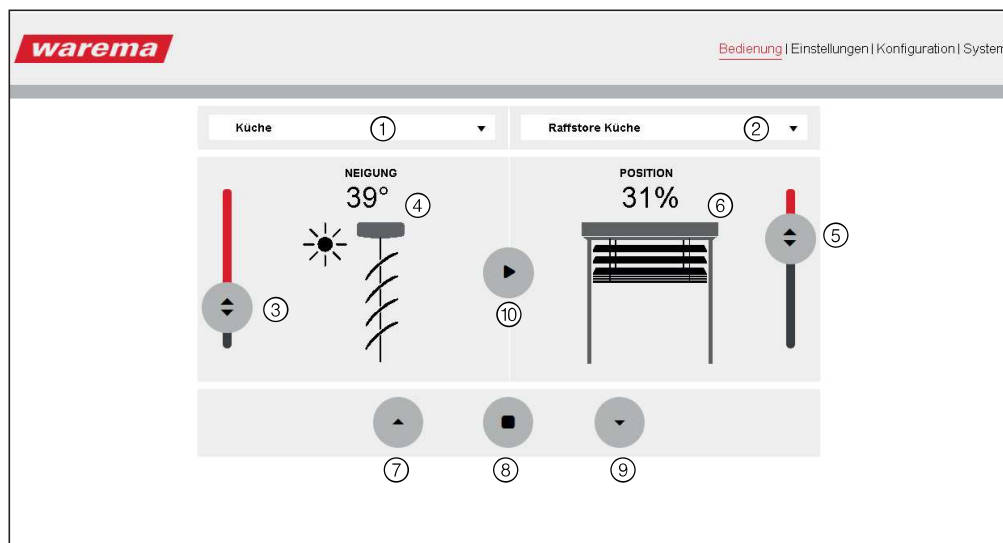
Abb. 8 Oberfläche des WAREMA climatronic® WebControl, Menü "Bedienung"
