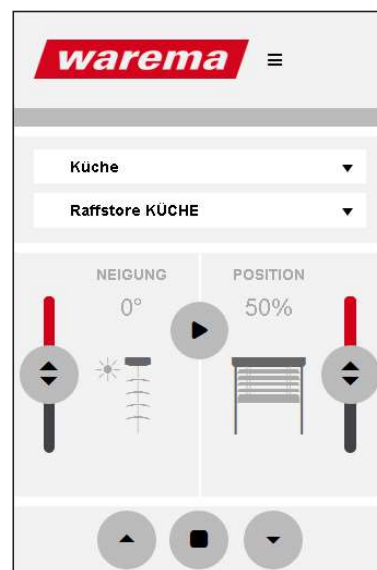
Abb. 6 Bedienoberfläche auf einem Smartphone
